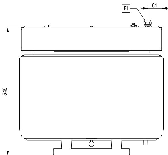
Boven aanzicht
